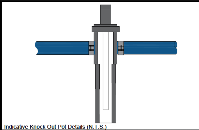
Indicative Knock Out Pot Details (N.T.S.)
